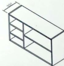
Wall unit 1050 X 300 X 600-2 QTY
